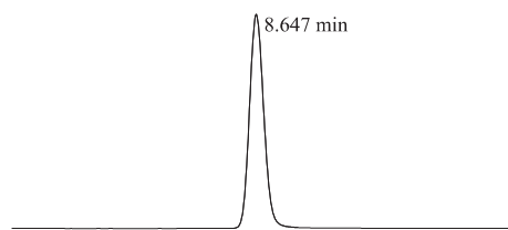
图1 丁香菌酯原药的高效液相色谱图
